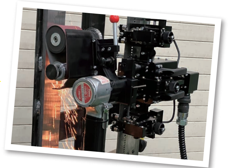
株式会社カットランドジャパン 溶接ビード自動研削機 SE・サンダー
